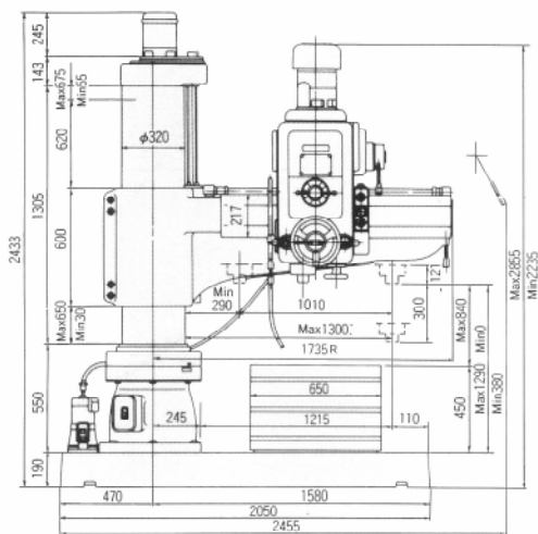
●外形図
